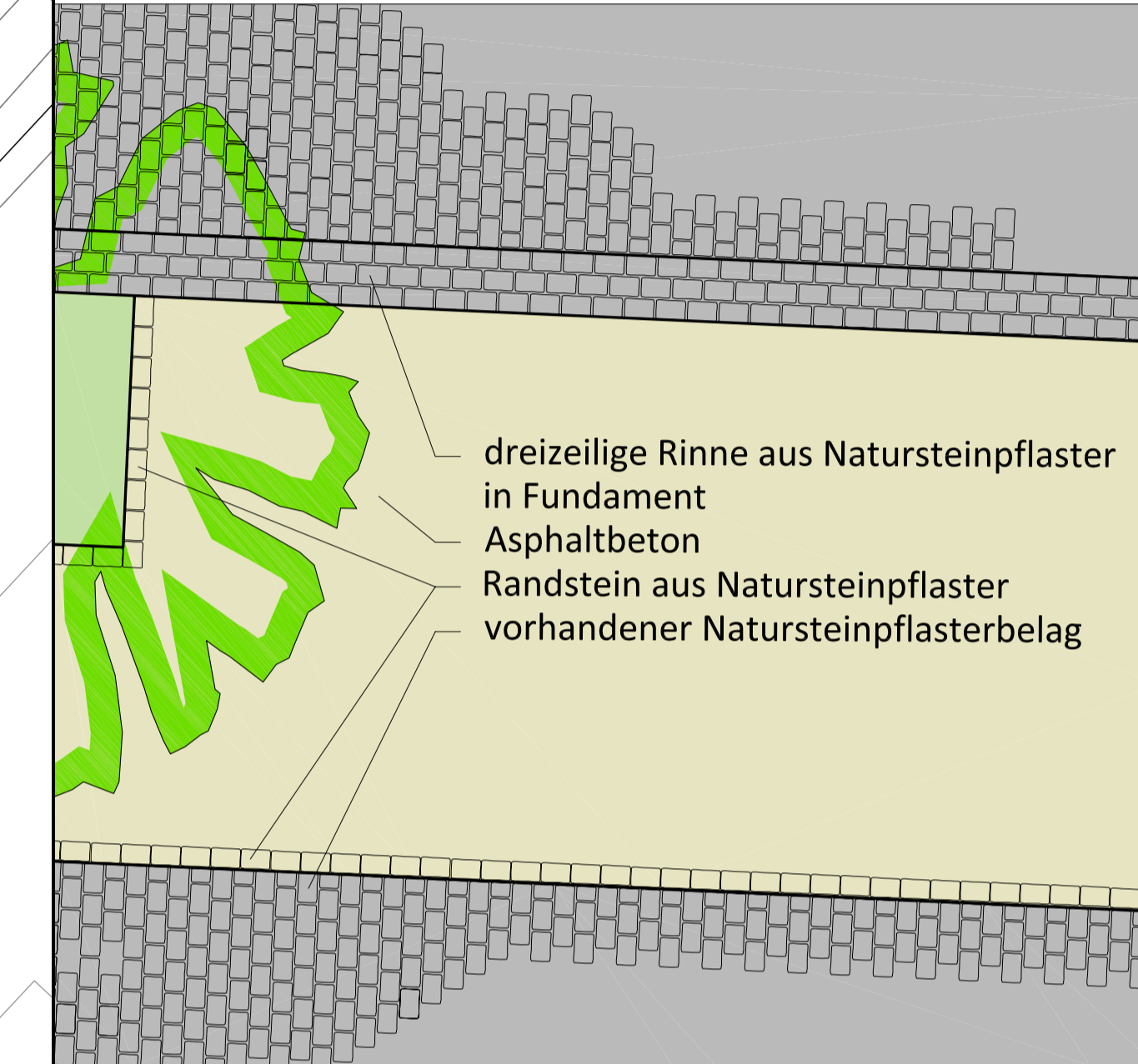
Detailausschnitt im M 1:20
