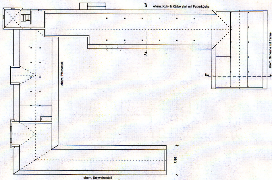
Dachgeschoss Bestand Maßstab 1:500
