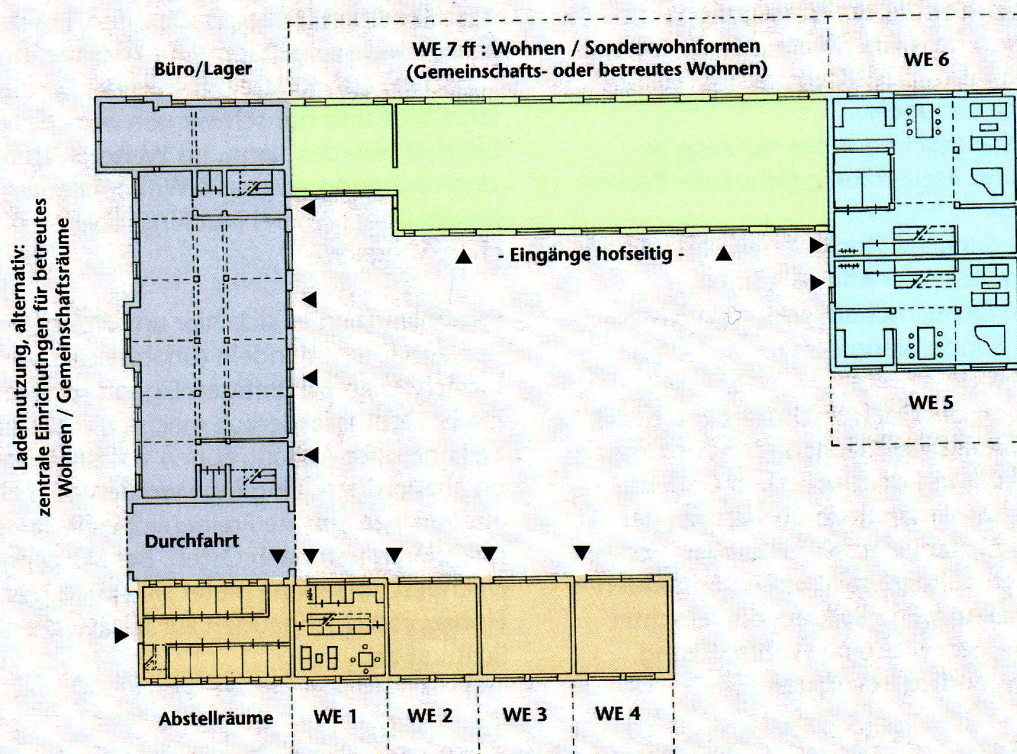
Erdgeschoss neu Maßstab 1:500
