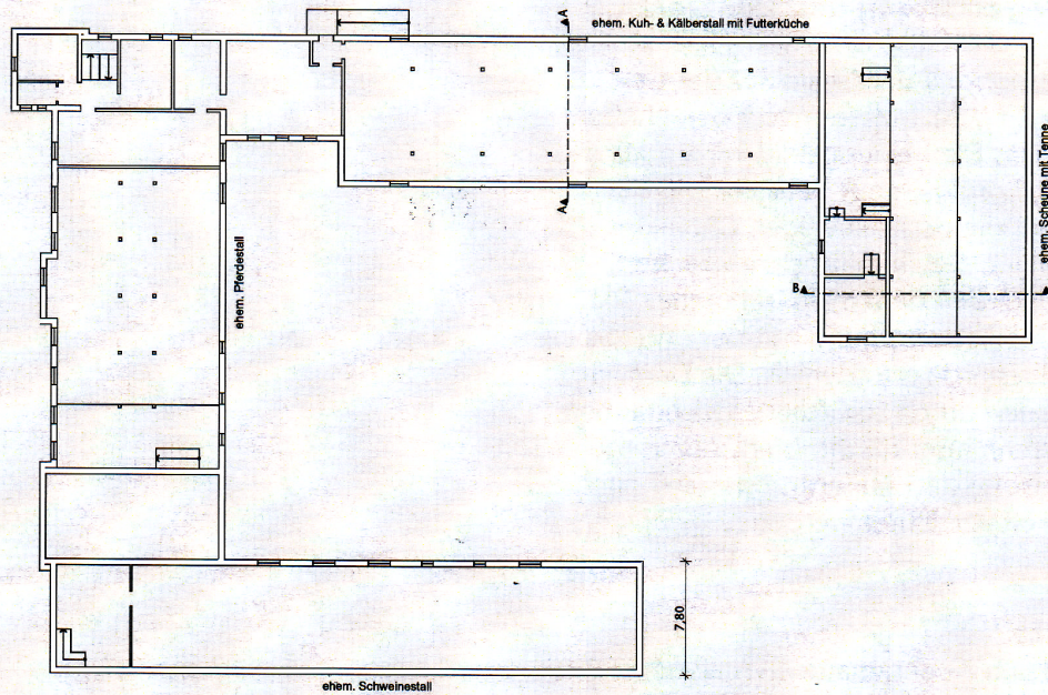
1. Obergeschoss Bestand Maßstab 1:500
