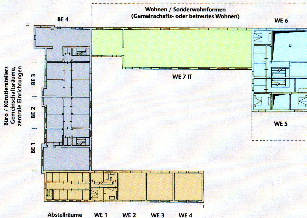
1. Obergeschoss neu Maßstab 1:500
