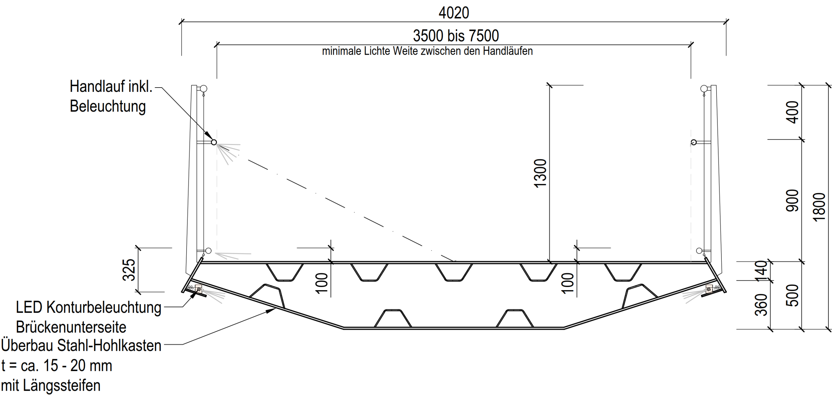
Regelquerschnitt - Loop
