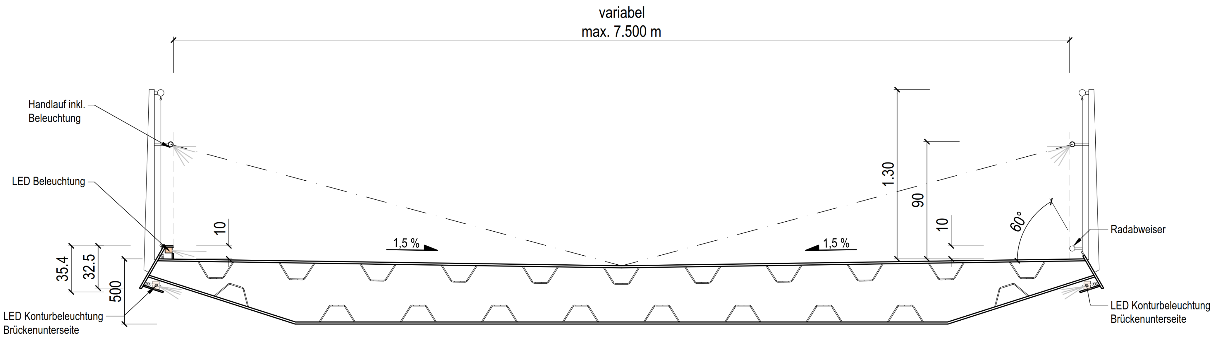
Regelquerschnitt - Brücke
